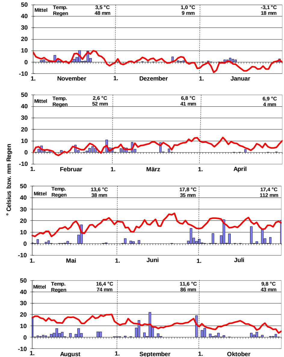
Witterungsverlauf am Standort Kyllburgweiler 2016/2017
