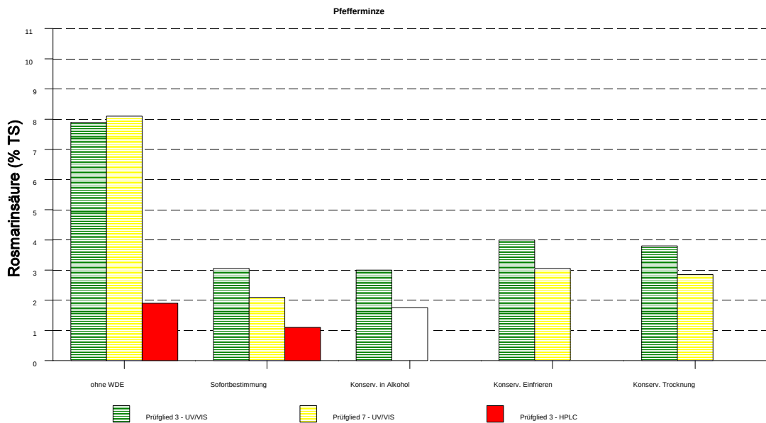
Abbildung 2: Rosmaringehalte von Pfefferminze vor und nach der Wasserdampfextraktion bei unterschiedlicher Konservierung
