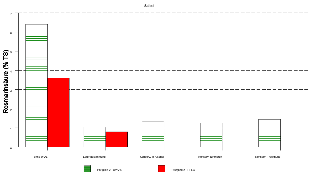
Abbildung 5: Rosmaringehalte von Salbei vor und nach der Wasserdampfextraktion bei unterschiedlicher Konservierung
