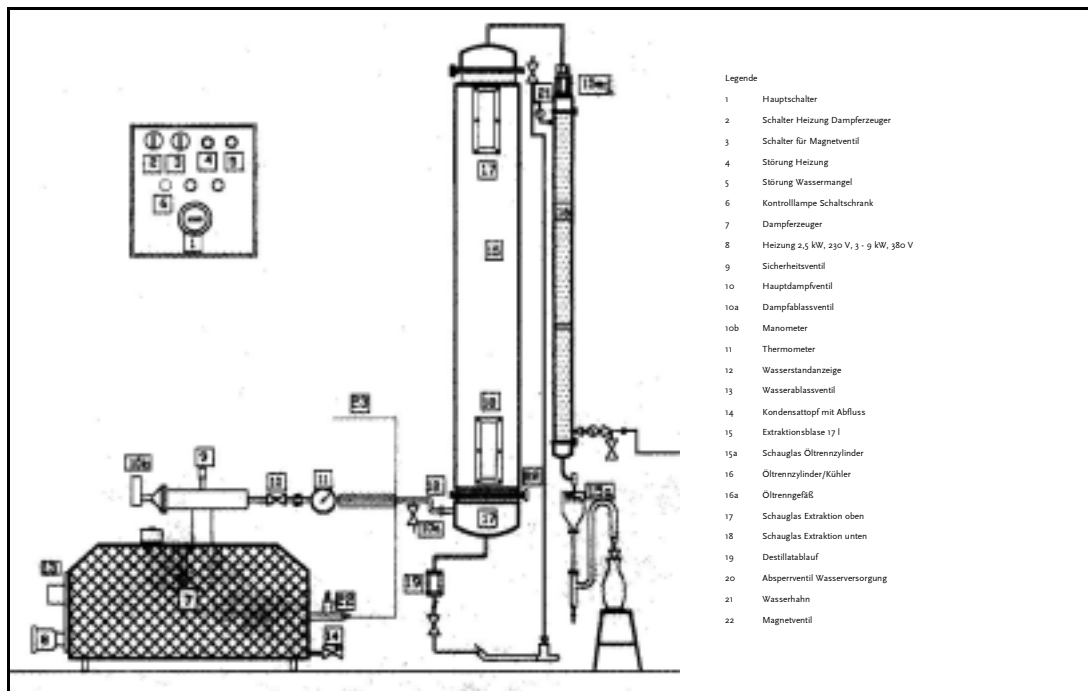
Abbildung 1: Aufbau der Wasserdampfextraktionsanlage
