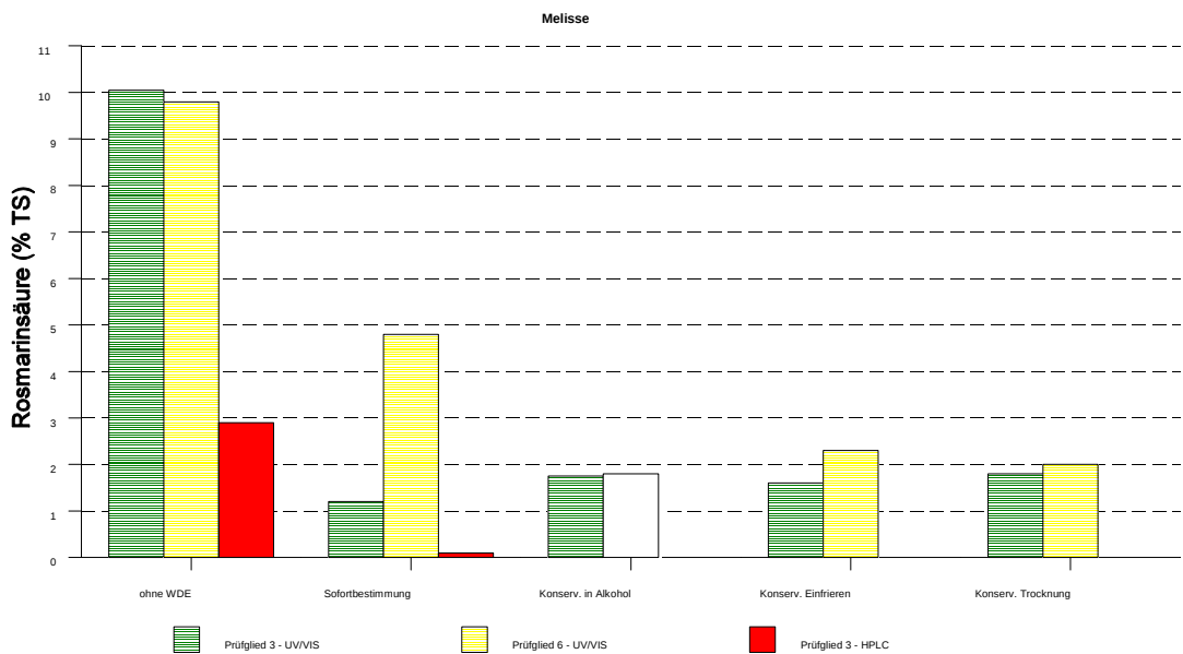
Abbildung 3: Rosmaringehalte von Melisse vor und nach der Wasserdampfextraktion bei unterschiedlicher Konservierung
