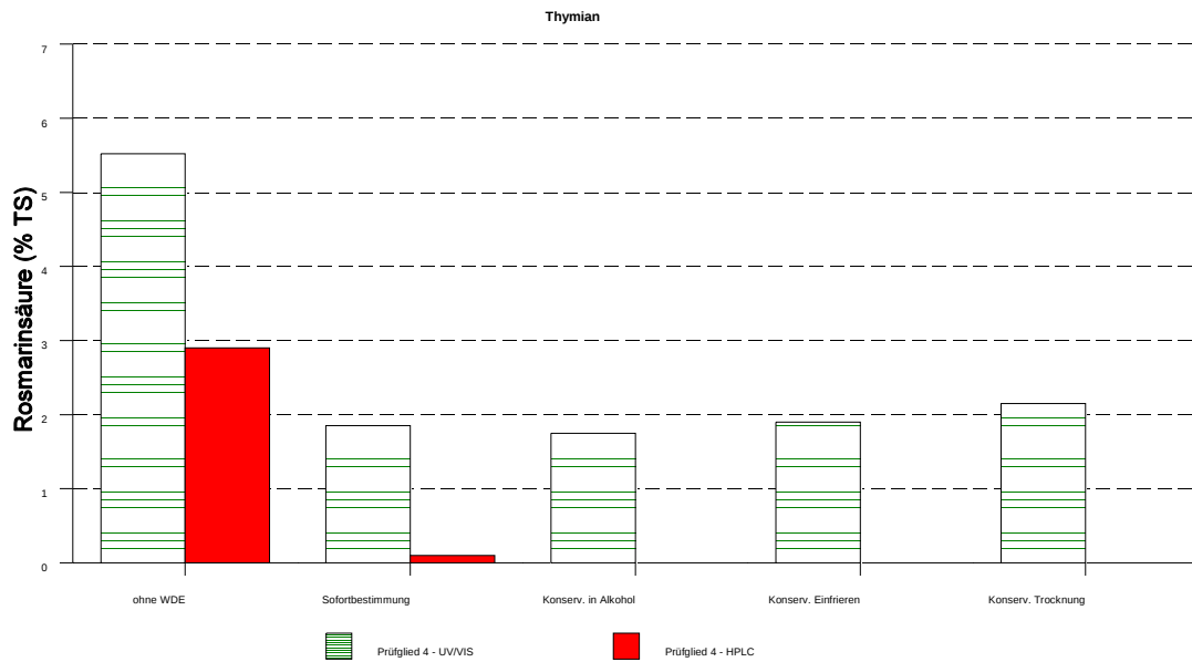
Abbildung 4: Rosmaringehalte von Thymian vor und nach der Wasserdampfextraktion bei unterschiedlicher Konservierung
