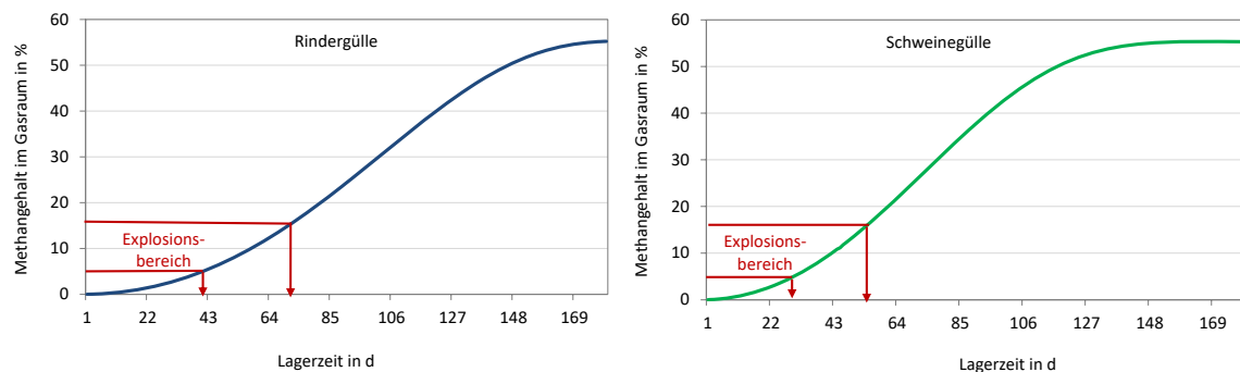
Abb. 6: Entwicklung der Methankonzentration für Rinder- und Schweinegülle bei der gasdichten Lagerung im Rundbehälter mit Doppelmembranhaut (Reinhold 2020). Zusätzlich ist der Bereich eingezeichnet, in dem das Gasgemisch explosionsfähig ist. Berechnung auf Basis der Emissionsinventare (Haenel et al. 2020).
