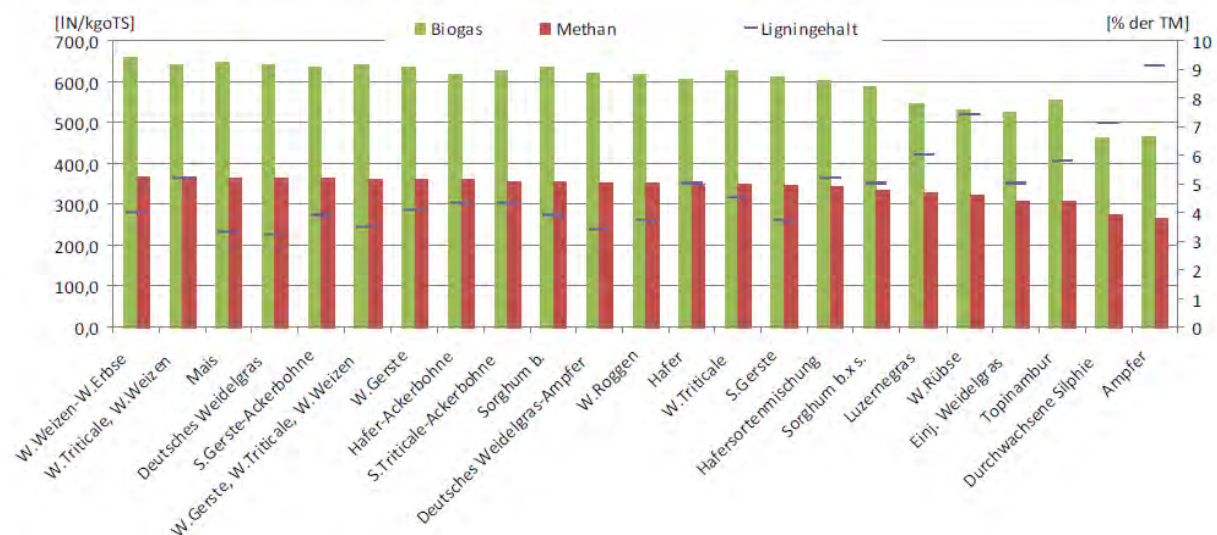
Abbildung 3: Spezifische Biogas- und Methanausbeuten sowie Ligningehalte aller bisher im HBT untersuchten Fruchtarten, nach absteigender Methanausbeute geordnet (n = 732)
