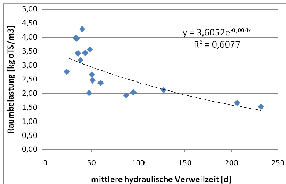
Abbil- 22: Zusammenhang zwischen Raumbelastung (in kg oTS/m 3 ) und Verweilzeit (in Tagen)
