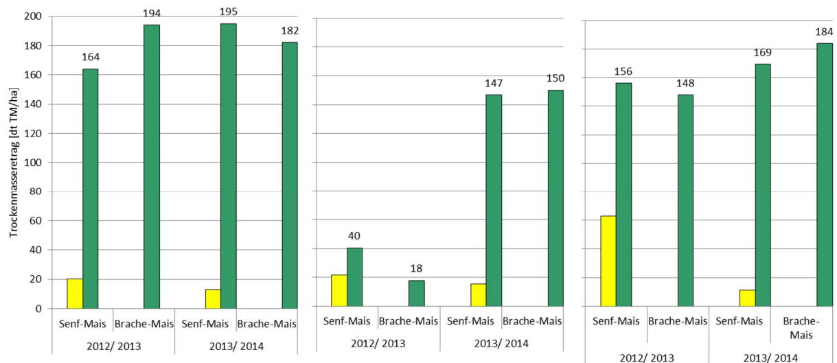
Abbildung 14: Trockenmasseerträge Mais nach ZwF Senf, im Vergleich zu Mais ohne ZwF, 2012 bis 2014, drei Standorte (von links nach rechts: Dornburg, Ascha, Werlte)
