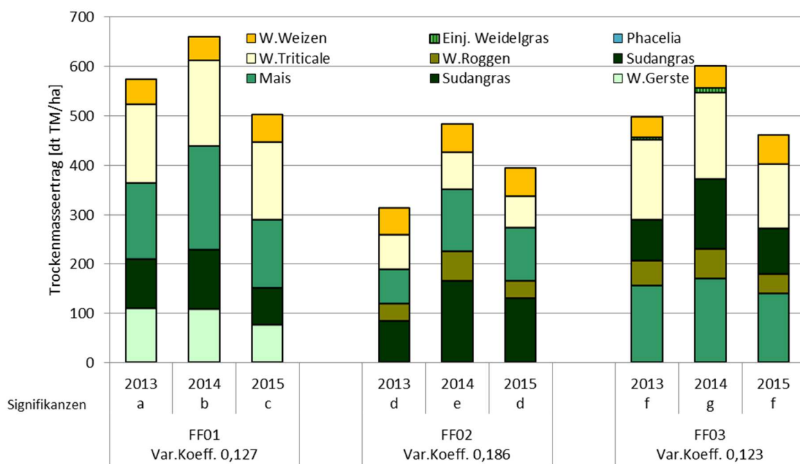
Abbildung 23: Trockenmasseerträge, Dornburg; 5. Anlage bis 8. Anlage; 2013 bis 2015; FF01 bis FF03; Signifikanzen für p \leq 0,05 ; Var.Koeff. der kumulierten Trockenmasseerträge zwischen den Jahren als Maßgröße der Ertragsvariabilität der FF-Leistung
