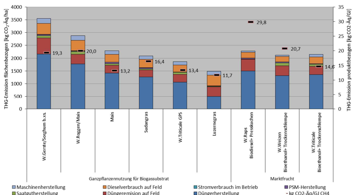
Abbildung 17: THG-Emission ausgewählter Energiepflanzen, Zweikulturnutzungssysteme und Marktfrüchte, Mittelwert 1. bis 4. Anlage (2005 bis 2013), Standort Dornburg
