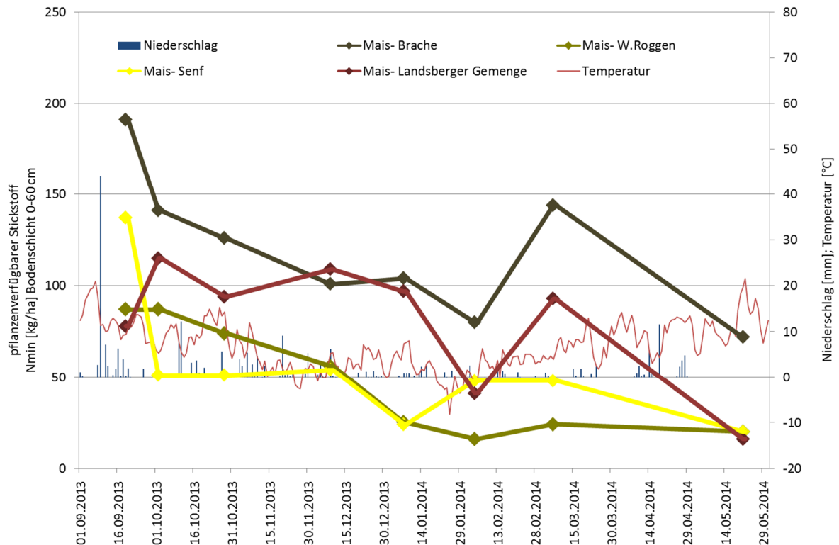
Abbildung 21: N_{\min} -Verlauf und Witterung unter verschiedenen Zwischenfrüchten nach Mais, Burkersdorf, September 2013 bis Juni 2014
