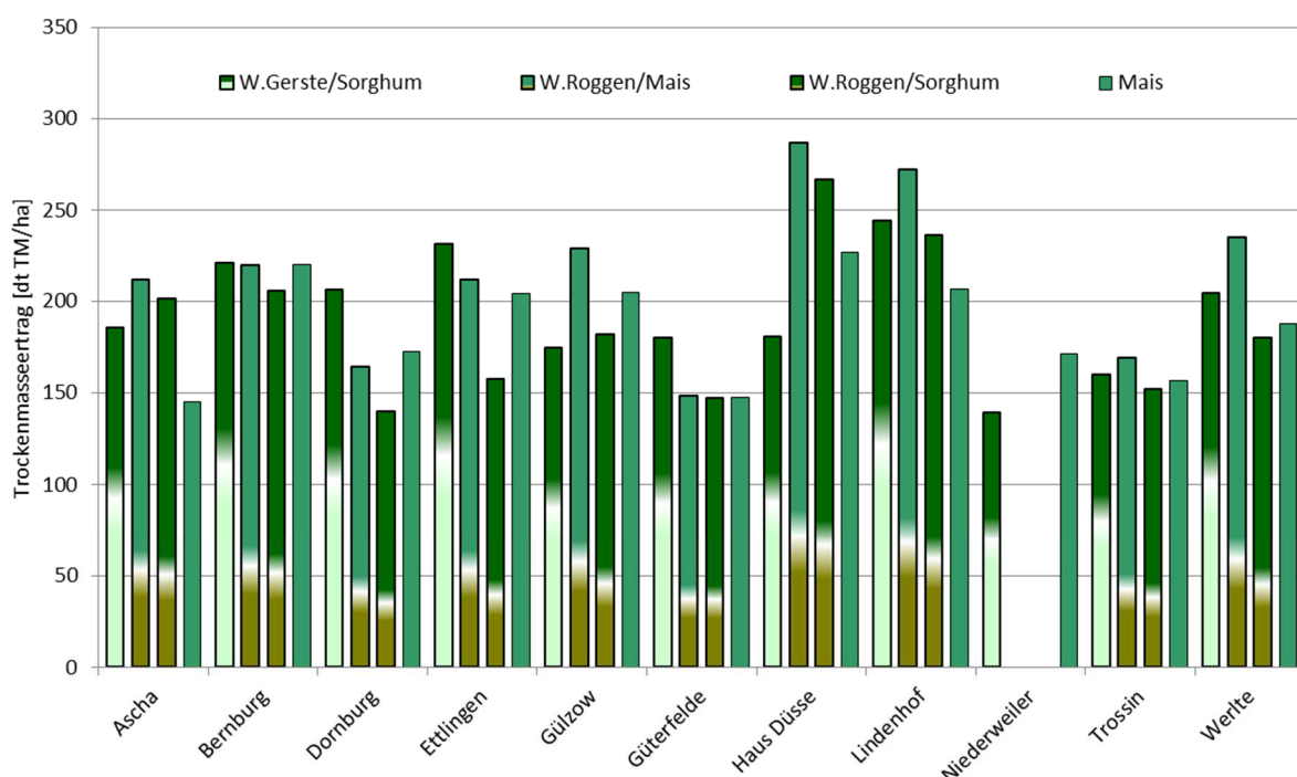
Abbildung 15: Mittlere Trockenmasseerträge Zweikulturnutzungssysteme und Mais (HF); alle Standorte, Grundversuch, 2005 bis 2015, n versuchsbedingt voneinander abweichend
