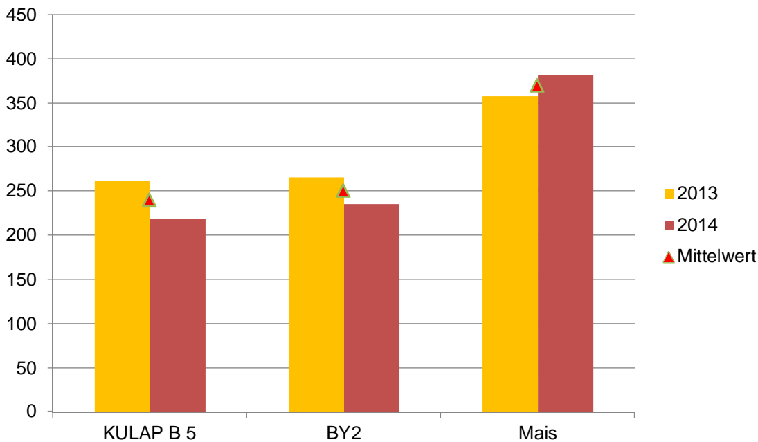
Abbildung 19: Methanausbeuten (NI/kg oTS) mehrjähriger Blühmischungen im Vergleich zu Silomais, VS Dornburg 2013 und 2014
