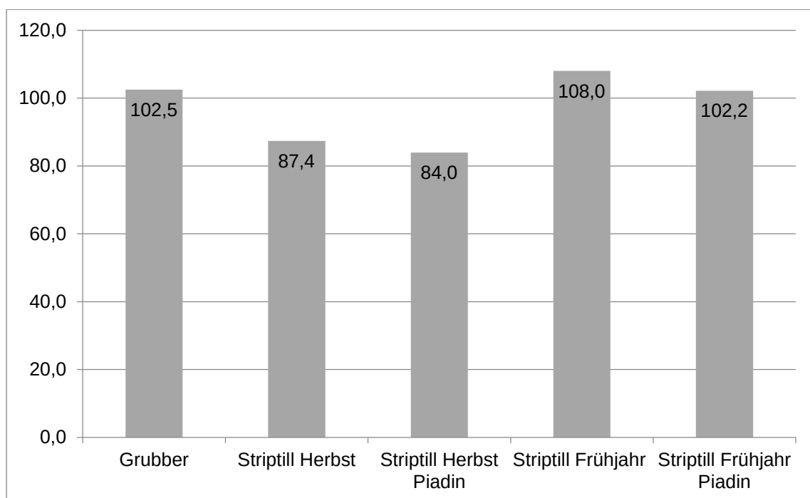
Abb. 5: Relativerträge in Prozent (Mittelwert über alle Jahre und Varianten= 100 %) bei Silomais 2014 bis 2016 (Piadin: Nitrifikationsinhibitor) (Grubber: Gärsubstratausbringung ganzflächig mit Grubbereinarbeitung; Strip-Till: Gärsubstratausbringung mit dem Strip-Till-Verfahren im Herbst bzw. im Frühjahr)
