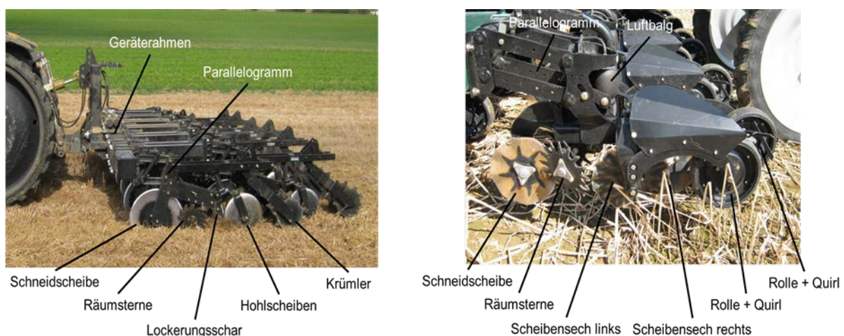
Bild 1: Streifenbodenbearbeitungsaggregate mit Zinken (links) und Schneidscheiben (rechts)
